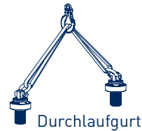
Durchlaufgurt
