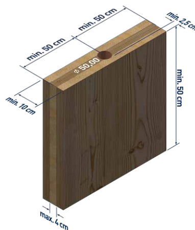
Manipulation verticale de bois contrecollé
