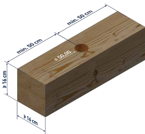
Manipulation horizontale de bois lamellé-collé et de bois massif
